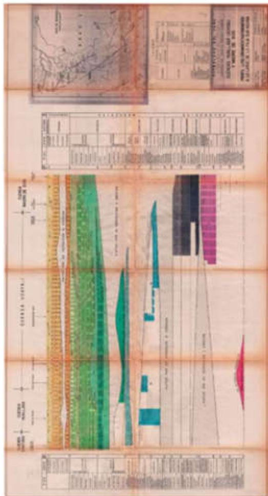
Figura 1. Esquema de correlación estratigráfica entre cuencas jurásicas y cretácicas (Santiago, Huallaga, Ucaiyali y Madera de Dios) que tiene como base del acervo bibliográfico elaborado por Hugo Valdivia en el año 1992.
